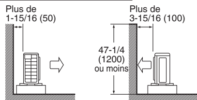
Vue latérale
