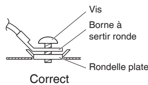
Sous-vue A
