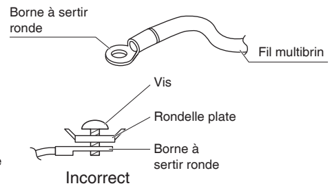
Sous-vue A
