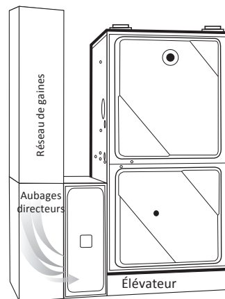
Élévateur du générateur d'air chaud
