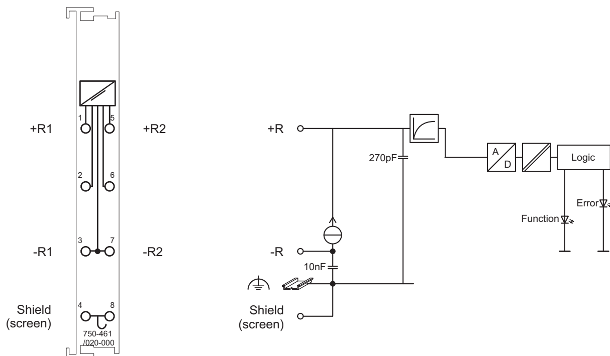
Fig. 2.1.3-3: 2-Channel Analog Input Module 750-461/020-000
